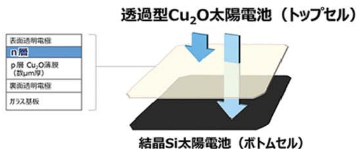
図1：開発したタンデム太陽電池の構成概略図
