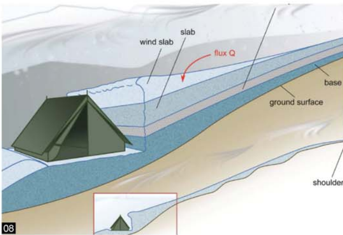
圖6 暴風雪中艱難前行的9位隊員 圖7 事發現場，被風雪壓扁了的帳篷 圖8 瑞士科學家根據資料模擬了當時營地的實況 圖9 瑞士科學家按照風速模擬突如其來的版塊雪崩對人體可能產生的巨大破壞，證明了隊員的死因並非源自野人或妖怪。
